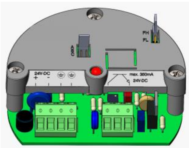
24V-DC mit Transistorausgang
